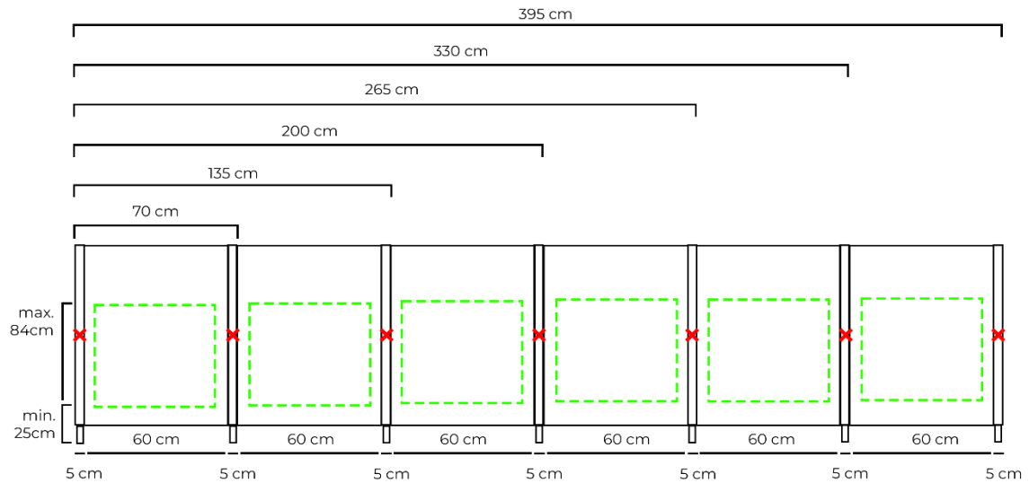
Figuur 1 Vooraanzicht buitenkeuken modules.
